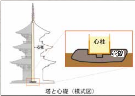
塔と心礎（模式図）
