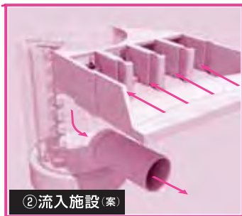
河川水を地下河川に流入させる施設を整備します。
