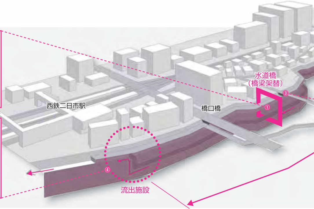
高尾川の地下10m程度に内径約5mの地下河川を整備します。
