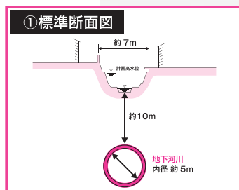
高尾川の地下10m程度に内径約5mの地下河川を整備します。
