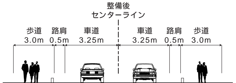
標準断面図 (幅員は現地にバラツキがあるため平均的な数値です)
