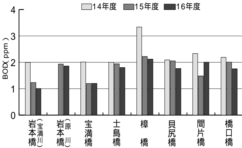
河川水質測定結果 (BOD) 平成14～16年度
