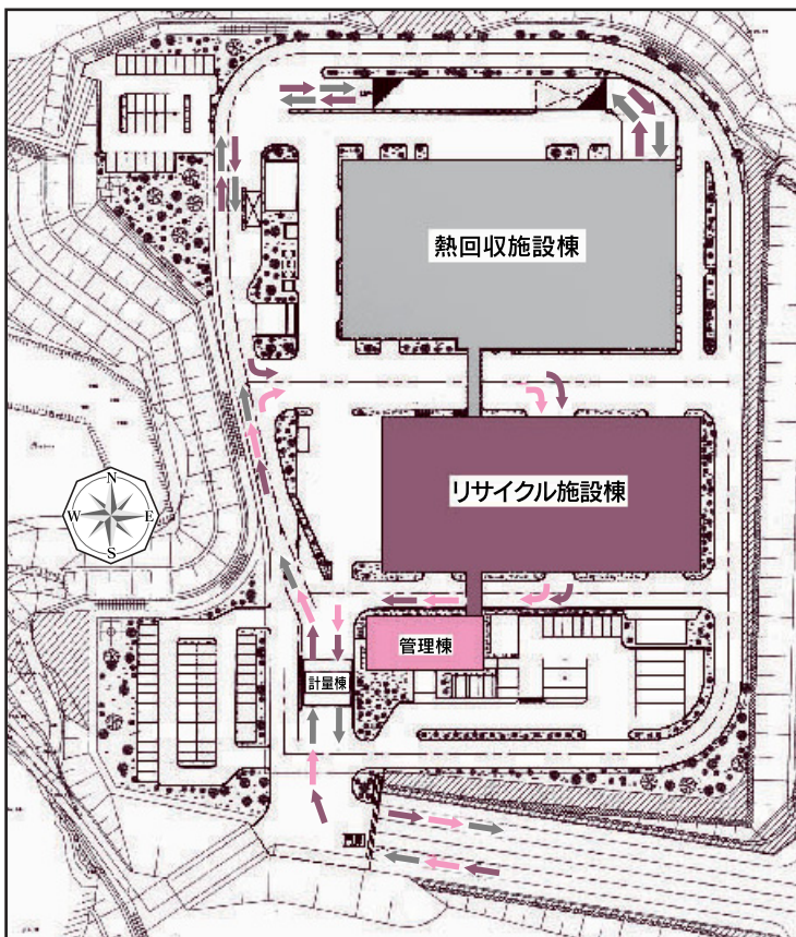
車両動線計画図
